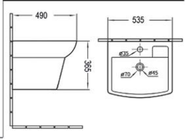
MODEL : 606 SIZE : 53.5X49X36.5 CM
